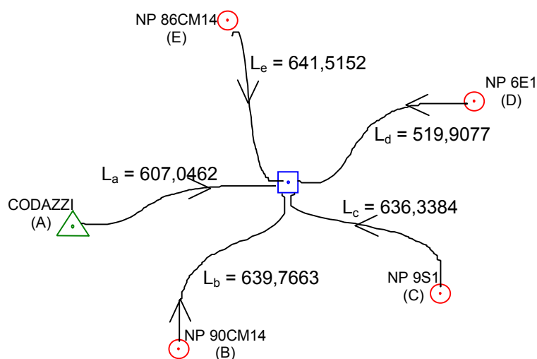
Figura 5. Representación esquemática de la determinación de la altura snmm de un punto a partir de información GPS y el modelo GEOCOL (Caso 1). El sentido de la flecha indica la altura mayor.
