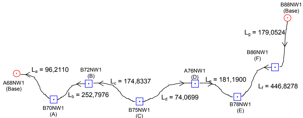
Figura 6. Representación esquemática de la determinación de la altura snmm de puntos contenidos en un perfil, a partir de información GPS y el modelo GEOCOL (Caso 2). El sentido de la flecha indica la altura mayor.
